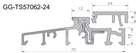
Próg COMBI 70 mm, 70 x 20 x 4500 mm, EV1, PCV szary, folia ochronna
