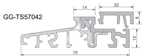
Próg ciepły ALU 70 mm, 70 x 20 x 4500 mm, EV1, PCV szary, folia ochronna
