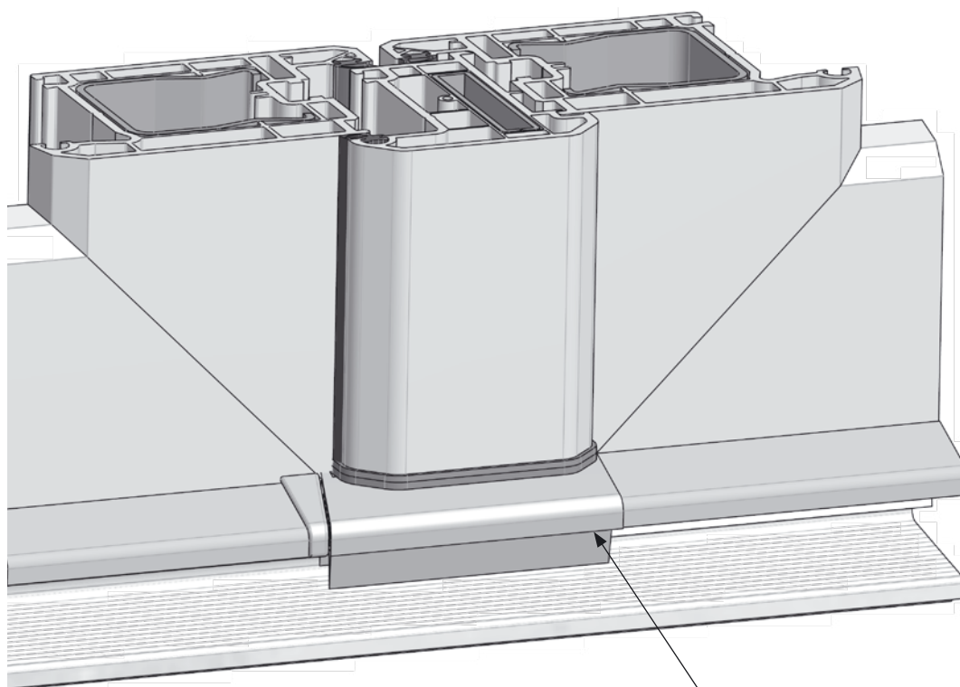
łącznik słupka ruchomego
