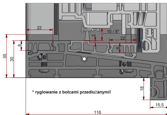
drzwi otwierane na zewnątrz
