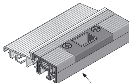
zaczep rygla drzwiowego z regulacją
